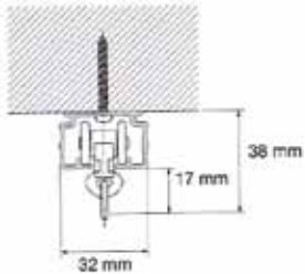
Fixation directe Suspendeur (00240011)
