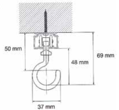
Fixation directe Suspendeur à crochet (00240056)
